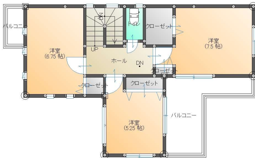
平面図-2F
